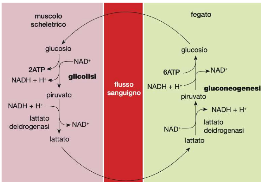
Figura 1 - Schema del ciclo di Cori che illustra i processi metabolici nel muscolo scheletrico (a sinistra) e nel fegato (a destra), collegati dal flusso sanguigno. FONTE: BioMicro, S. Recchia, A. De Benedictis, Lucisano Editore, pag 199.
